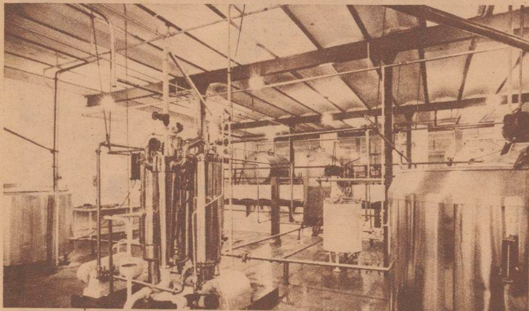
Sala de pasteurización, sistema Vacreador, único existente en España.
