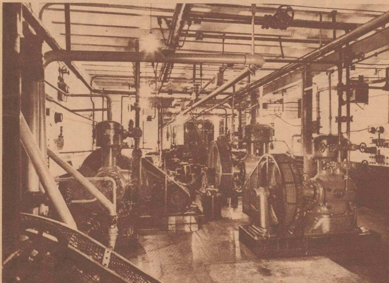
Un aspecto de la sala de compresores frigoríficos.
