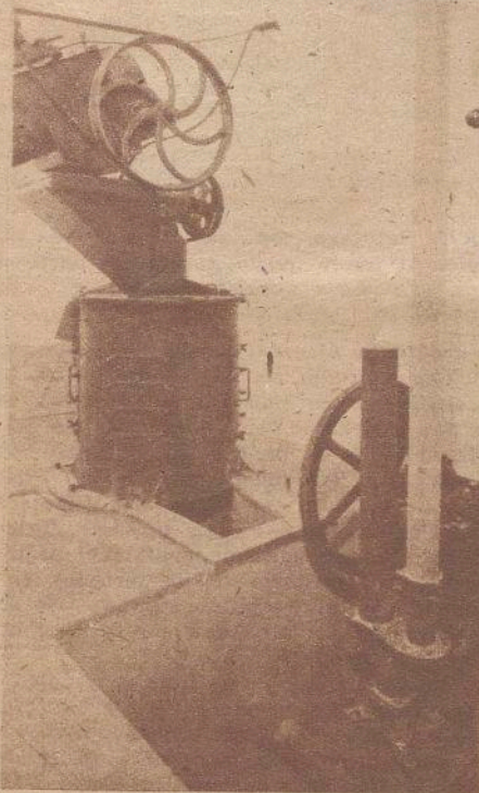
Superestrujadora centrífuga separadora de escobajo. Bomba de vendimia elevadora.
