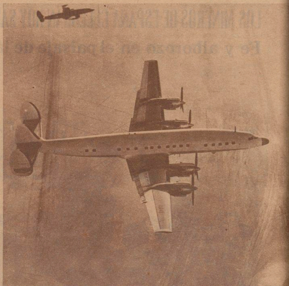
LAS ALAS MAYORES DEL MUNDO. —El Lockheed Super-Constellation 1649 es avión cuyas alas tienen mayor envergadura: 43,70 metros. El modelo posee una autonomía de diez mil kilómetros y empezará a prestar servicios comerciales en la próxima primavera. Cinco compañías aéreas han solicitado ya cuarenta y cuatro aviones de este tipo.
