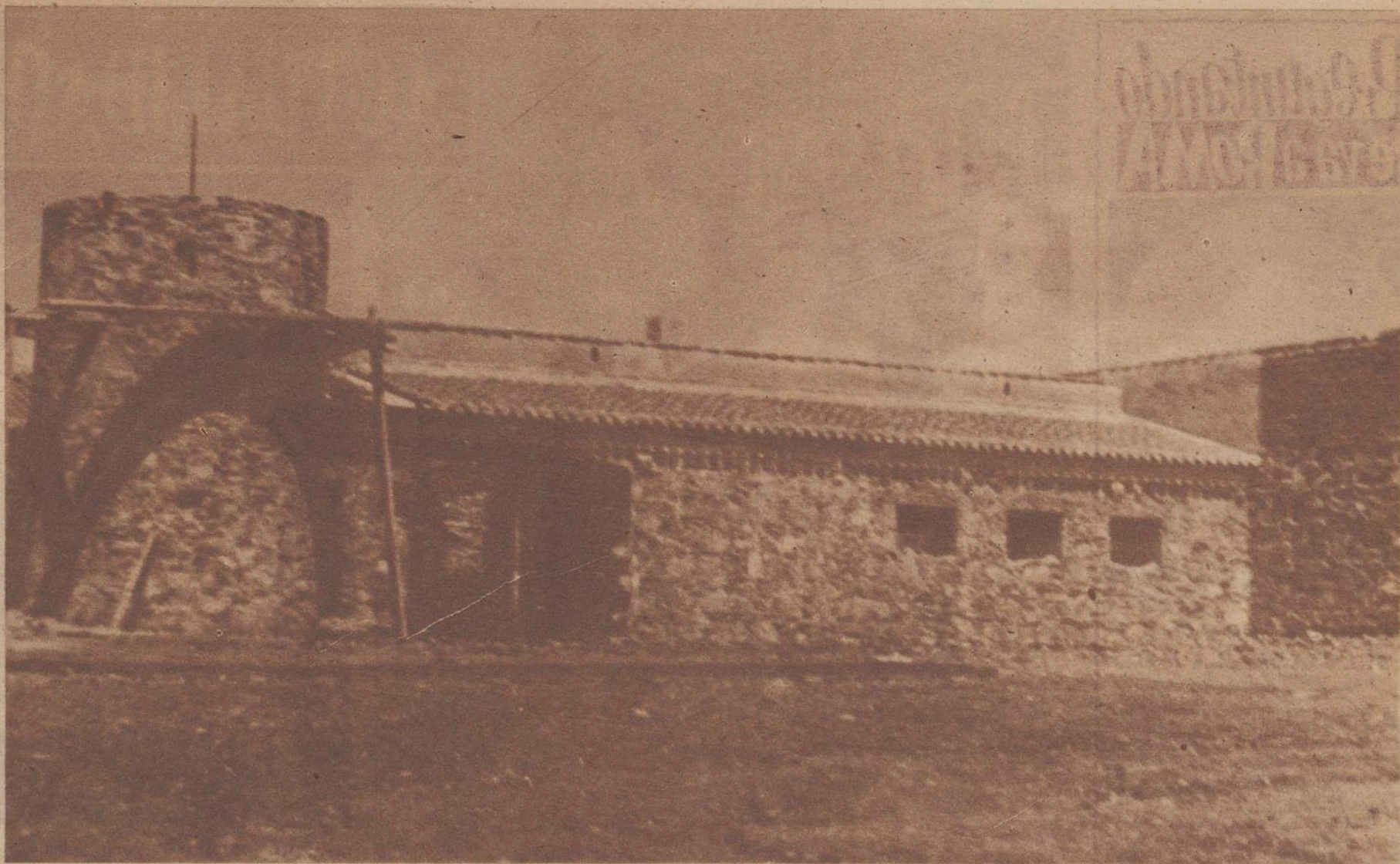
Vista del torreón para el transformador, y una vivienda adjunta para los colonos.
