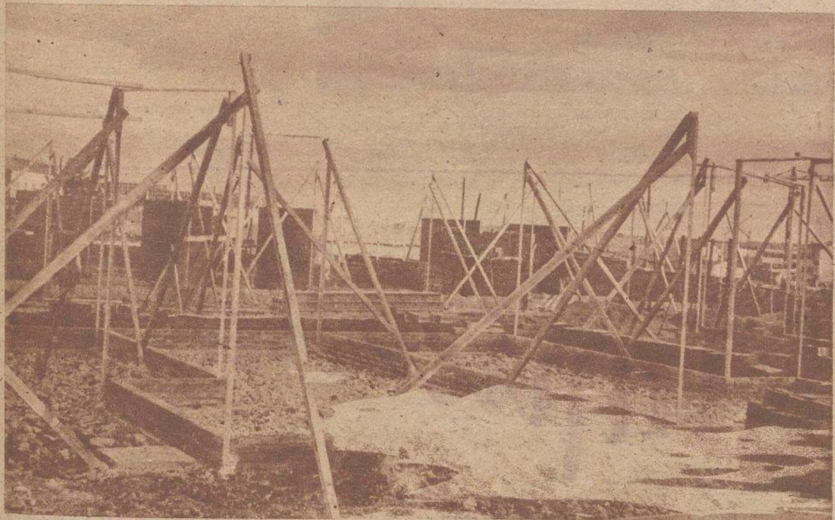
Nuevos procedimientos de trabajo hacen posible que se trabaje a la vez en todas las paredes maestras de estas casas. El cartel de cada una de las empresas concursantes anuncia un plazo mínimo de conclusión. Nuestra fotografía muestra cómo se las arbitran los albañiles para conseguir la vertical en los vértices y en las paredes laterales de cada una de las escuadras.—Fotos Porras.
